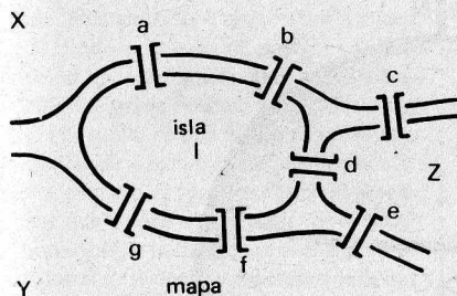
Problema de los puentes de Königsberg
