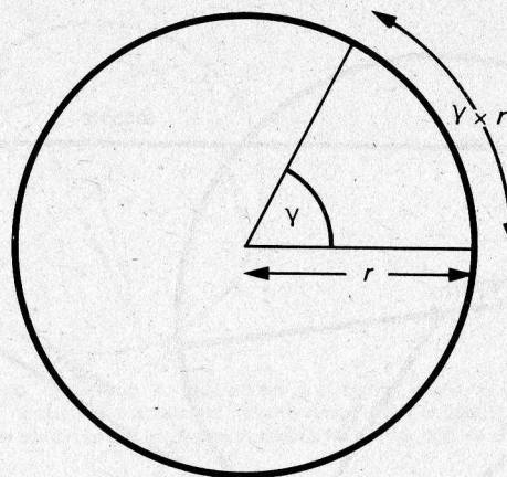
La medida circular: en un círculo de radio r y circunferencia 2\pi r , el ángulo \gamma radianes subtende un arco de longitud \gamma \times r .
