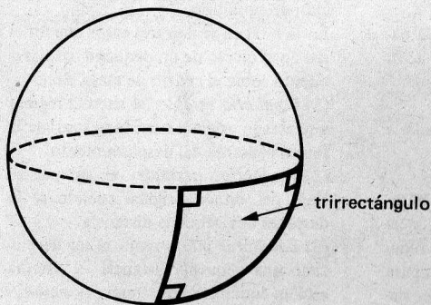
triángulos esféricos
