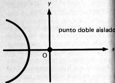
Cuatro tipos de punto doble en el origen de un sistema bidimensional de coordenadas cartesianas.
