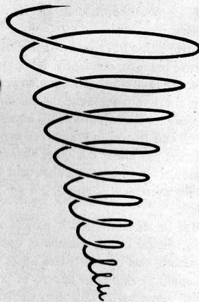
Hélice cónica
