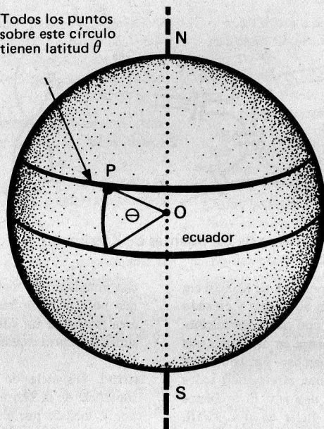
La latitud \theta de un punto P sobre la superficie de la Tierra.
