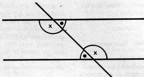
Ángulos alternos formados por una recta que corta a dos paralelas.
