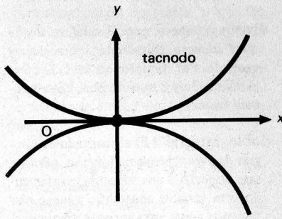
Cuatro tipos de punto doble en el origen de un sistema bidimensional de coordenadas cartesianas.
