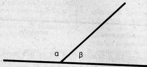
Angulos suplementarios: \alpha + \beta = 180^\circ
