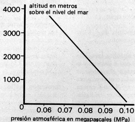
Gráfico de conversión para averiguar la altitud a partir de medidas de la presión atmosférica. (Presión atmosférica normal al nivel del mar: 1,01325 millones de pascales.)
