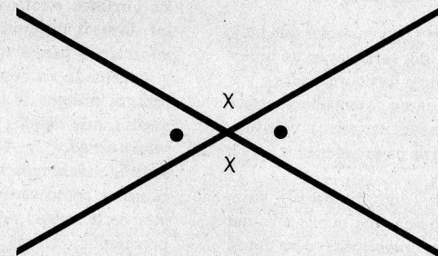
Ángulos opuestos por el vértice en la intersección de dos rectas.
