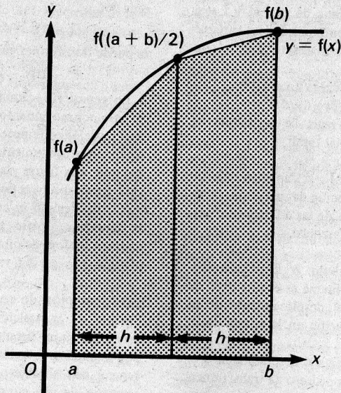
Aproximación por la regla del trapecio del área bajo una curva y = f(x) utilizando dos columnas en el intervalo x = a a x = b .
