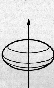
elipsoide achatado
