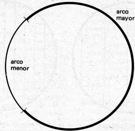
Arco: arcos mayor y menor de un círculo.
