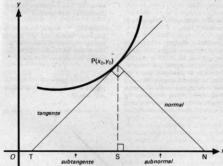
La subtangente TS y la subnormal SN de una curva en un punto P(x_0, y_0) .
