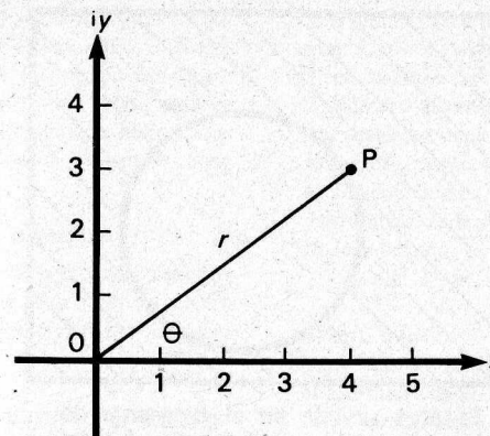
El punto P(4, 3) en un diagrama de Argand representa el número complejo z = 4 + 3i . En forma polar es z = r(\cos \theta + i \sin \theta) .
