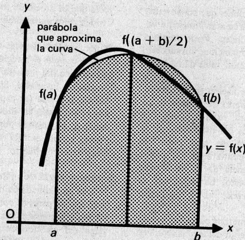
Aproximación por la regla de Simpson del área bajo una curva y = f(x) , utilizando dos columnas en el intervalo x = a a x = b .
