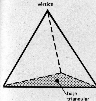
Pirámide triangular
