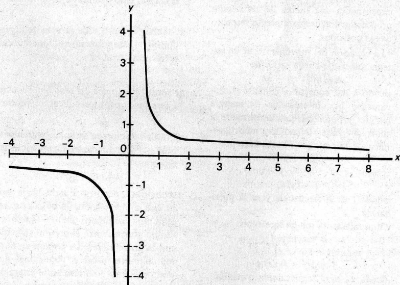
El eje x y el eje y son asíntotas de esta curva.
