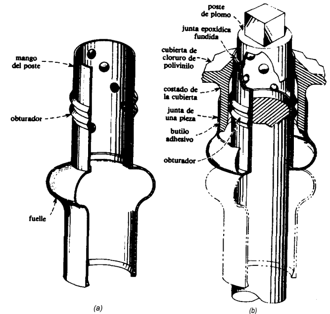
Fig. 8.22. Ensamblaje final después del sellado: (a) junta hermetica del poste de una pieza, (b) ensamblaje de la junta hermetica del poste.
