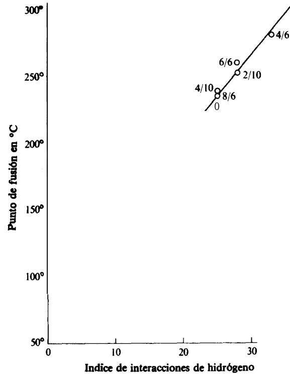
Fig. 8.15. Variación del punto de fusión en función del índice de interacciones de hidrógeno en los poliamidos con grupos pares de CH 2 .
