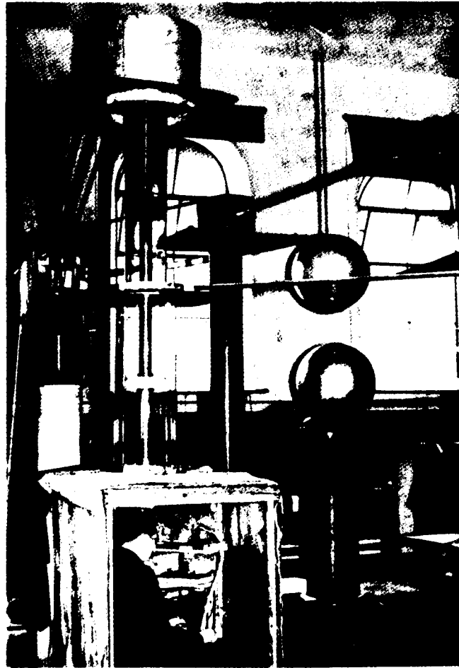
Fig. 9.6. Aparato de Cockcroft-Walton, con el cual se produjeron por primera vez partículas de alto voltaje para desintegrar artificialmente el núcleo atómico.
